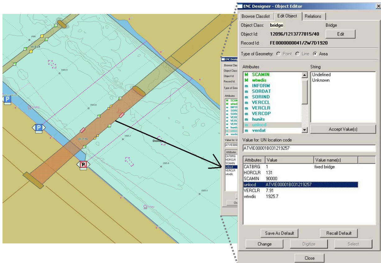
Figure 6 Brug-object in een Inland ENC
